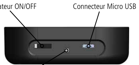
Figure 4 : Vue dessous
